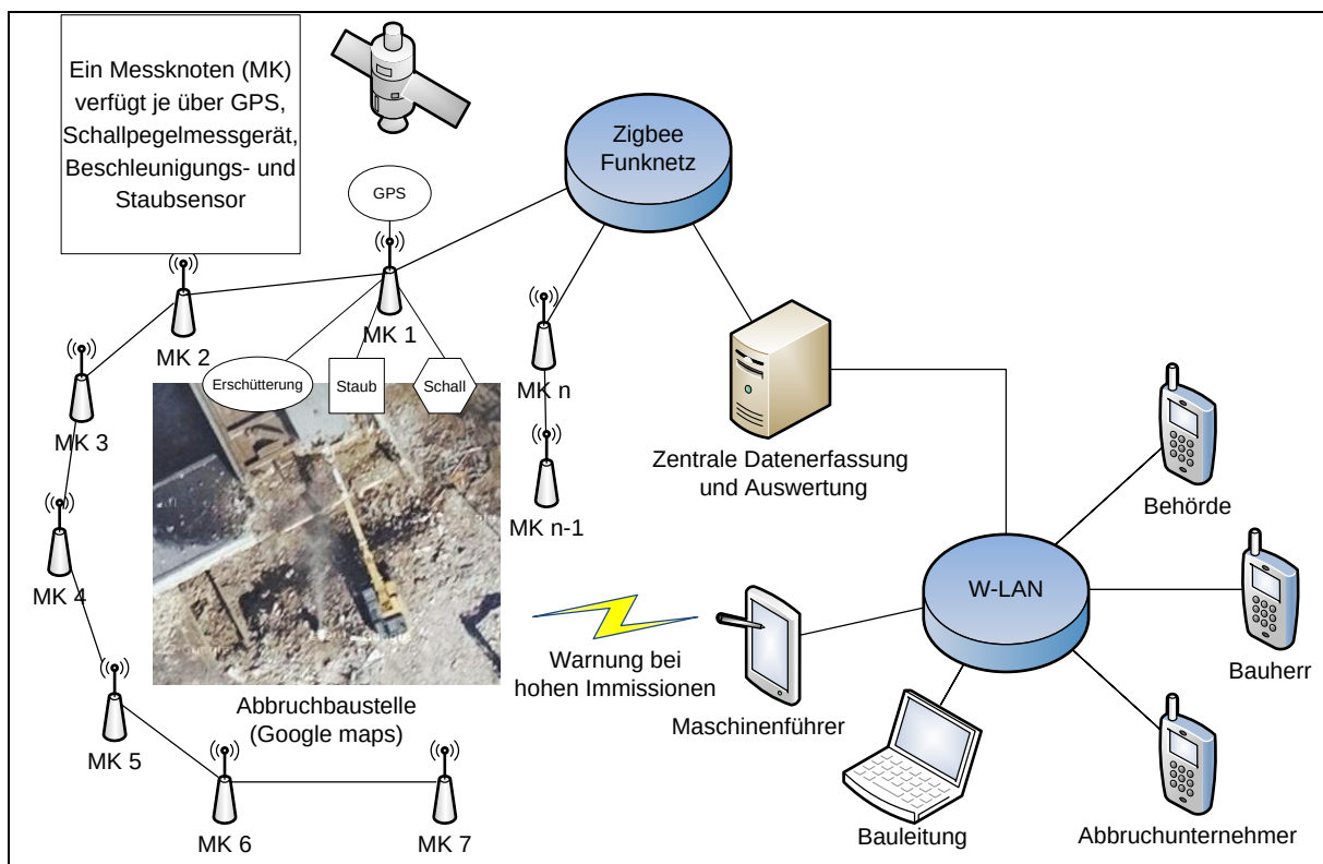
Abbildung 27: Aufbau des Immissionserfassungssystems
