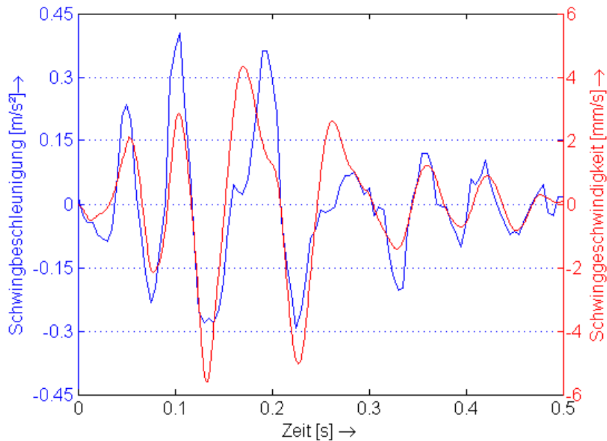
Abbildung 20: Zeitverlauf der Schwinggeschwindigkeit und -beschleunigung am Messpunkt 4 bei 21,45m Fallhöhe
