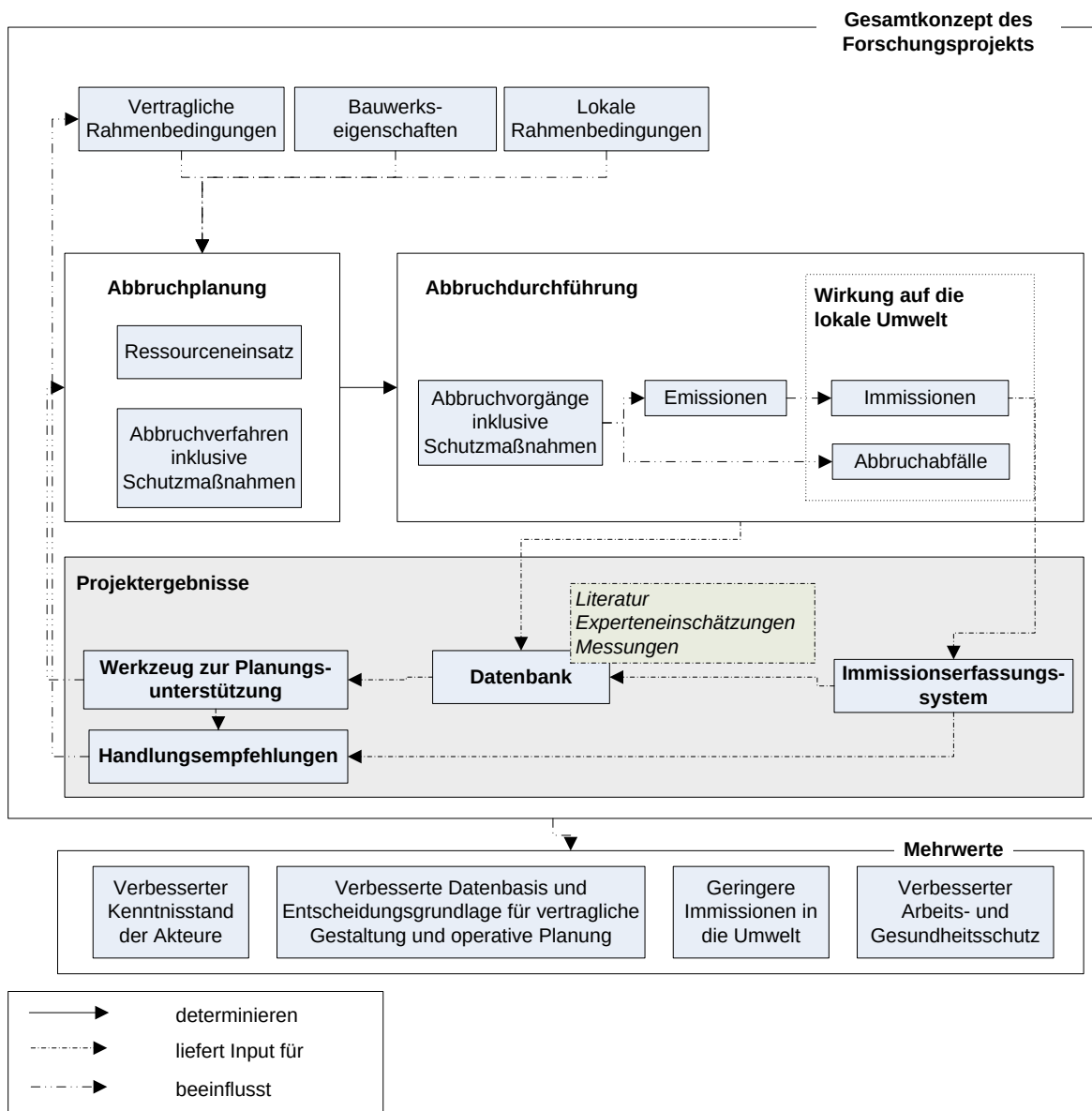
Abbildung 6: Gesamtkonzept des Forschungsprojekts
