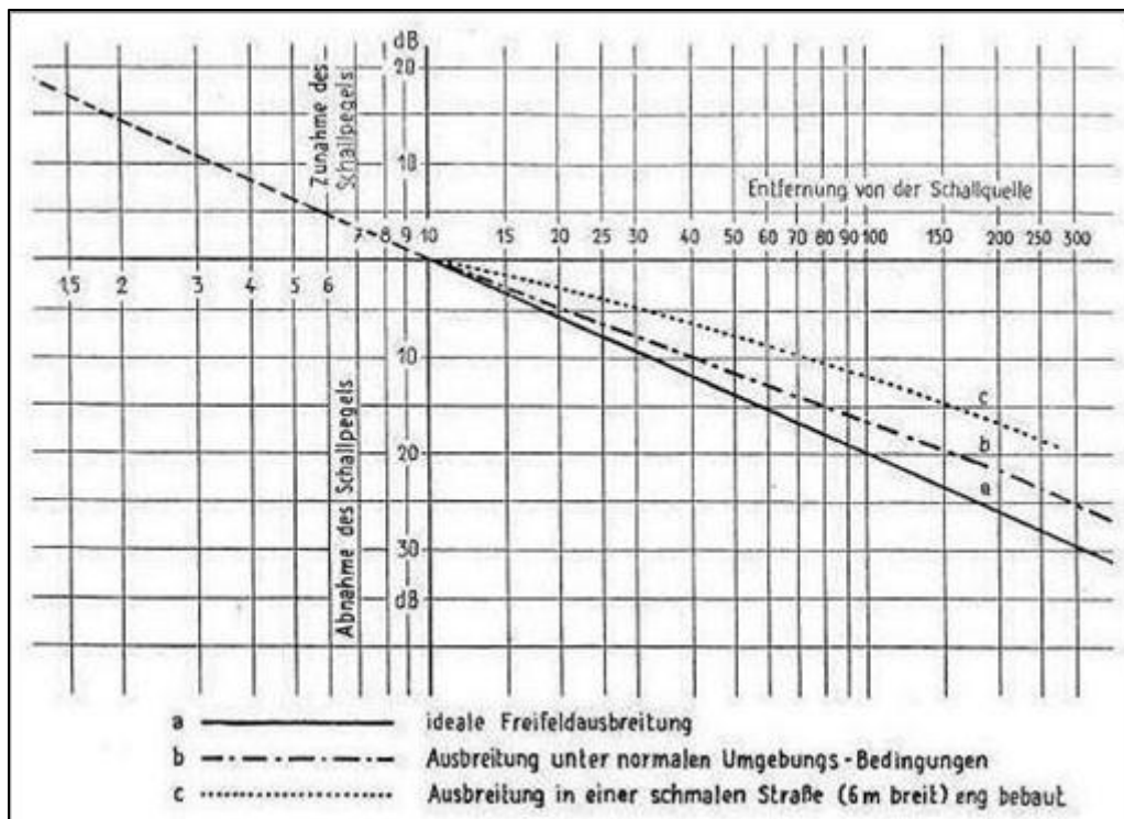
Abbildung 21: Änderung des Schalldruckpegels in Abhängigkeit von der Entfernung bezogen auf einen Schalldruckpegel in 10 m Entfernung (AVV Baulärm, 1970)
