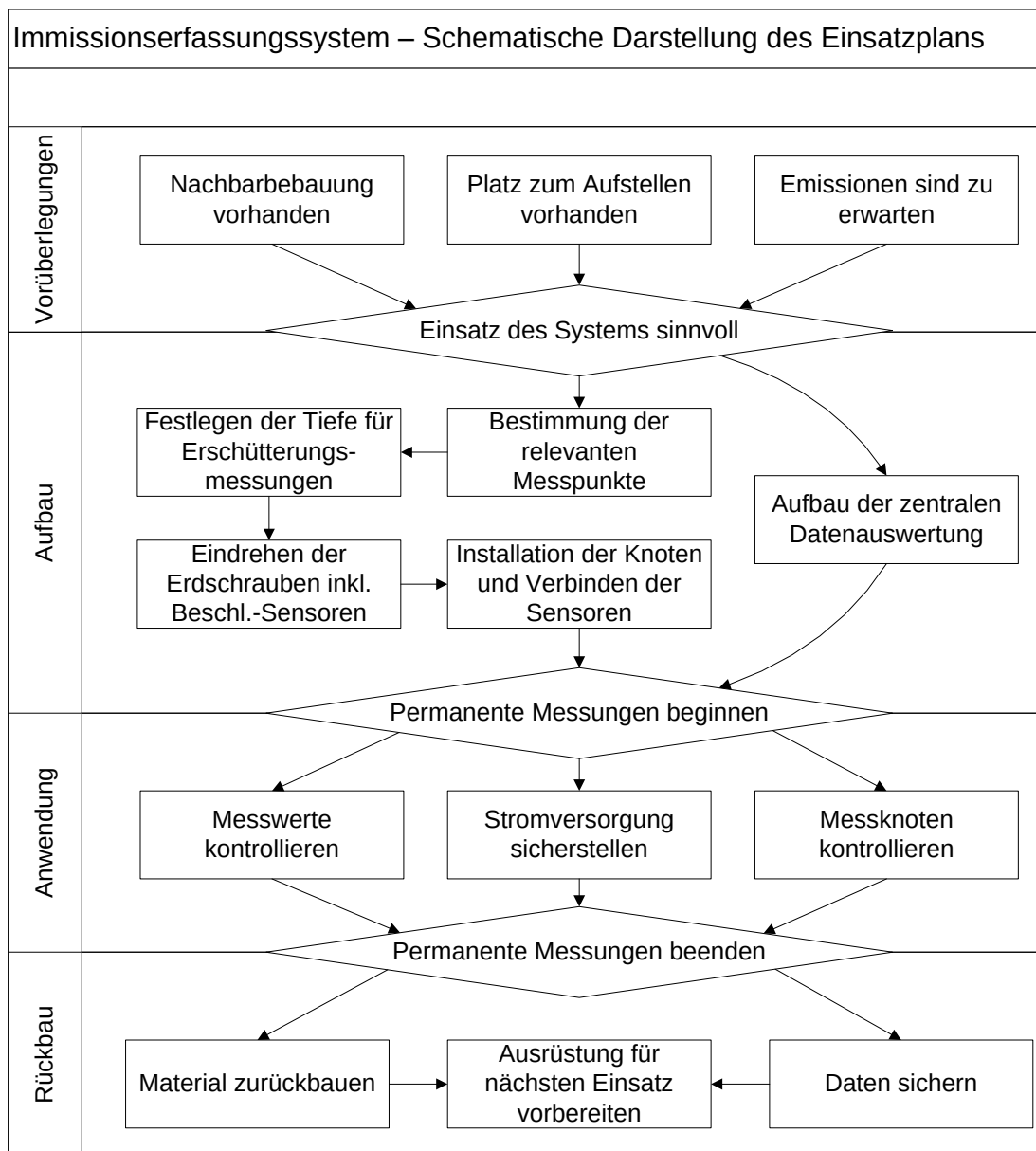
Abbildung 29: Abfolge des Einsatzes des Immissionserfassungssystems
