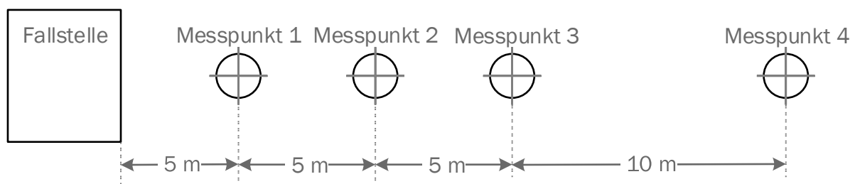
Abbildung 18: Messaufbau der Beschleunigungssensoren für die Fallversuche
