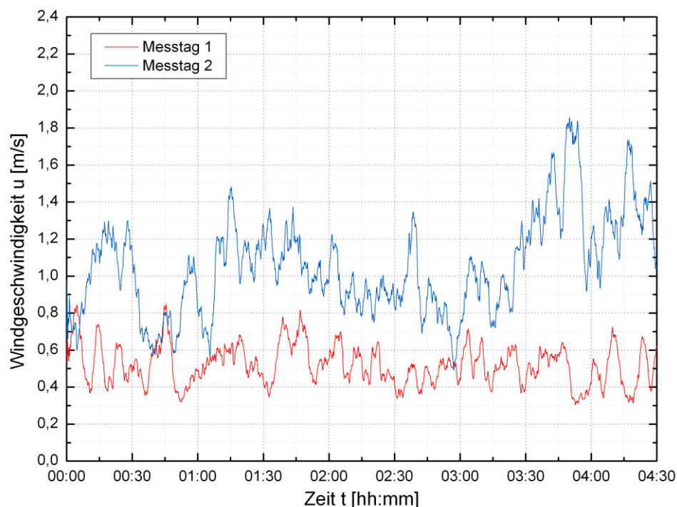
Abbildung 30: Windgeschwindigkeiten am 1. und 2. Messtag (ILK Dresden (2013))
