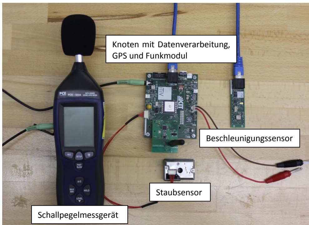
Abbildung 24: Sensorknoten und Schallpegelmessgerät
