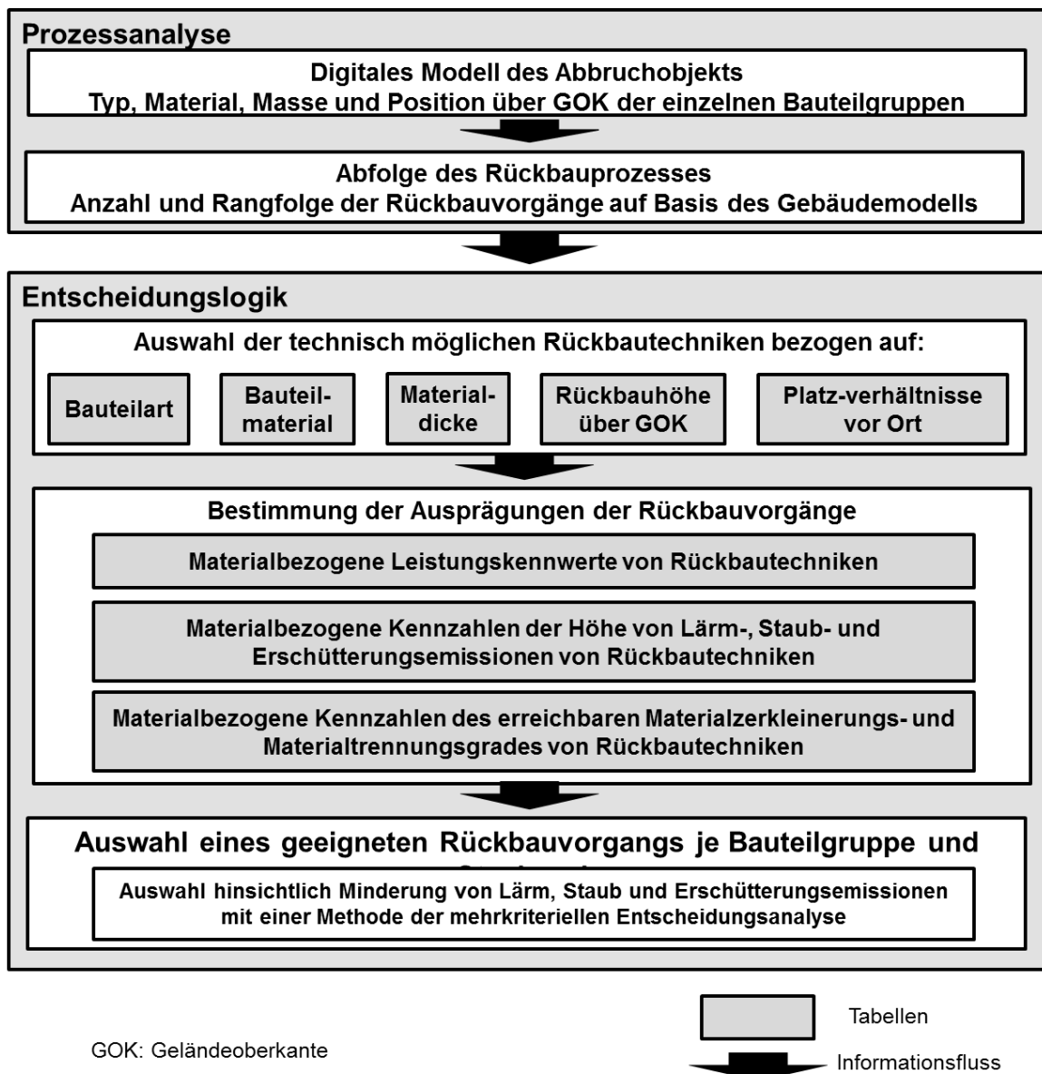
Abbildung 8: Prozessanalyse und Entscheidungslogik
