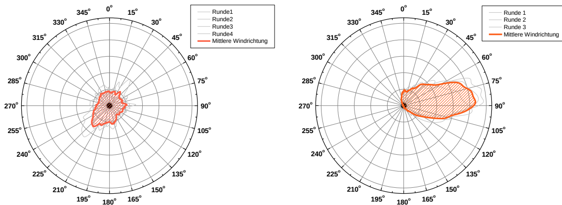
Abbildung 31: Windrichtungen am 1. (links) und 2. (rechts) Messtag (ILK Dresden (2013))
