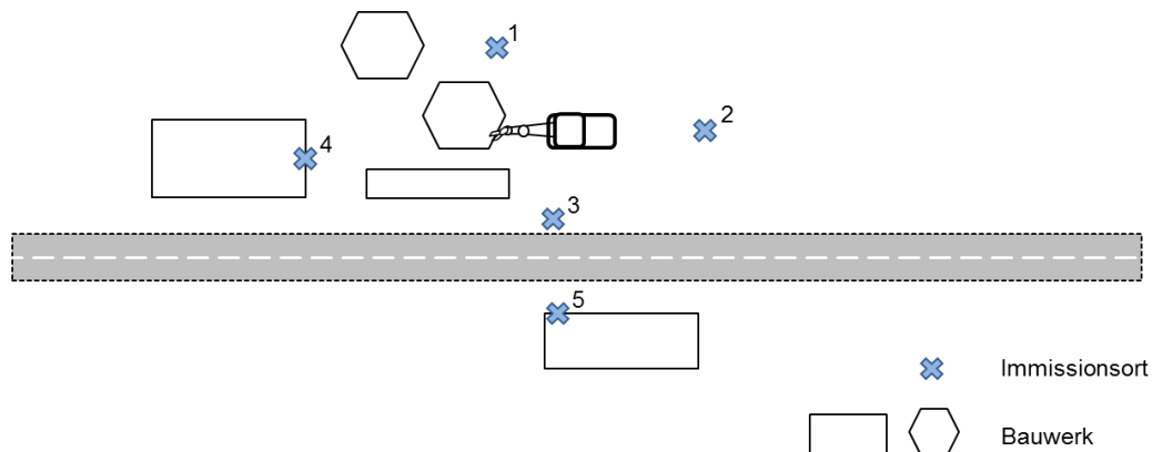
Abbildung 4: Mögliche Messpunkte für die Ermittlung von Staubdeposition und Feinstaub (PM10) (Draufsicht)
