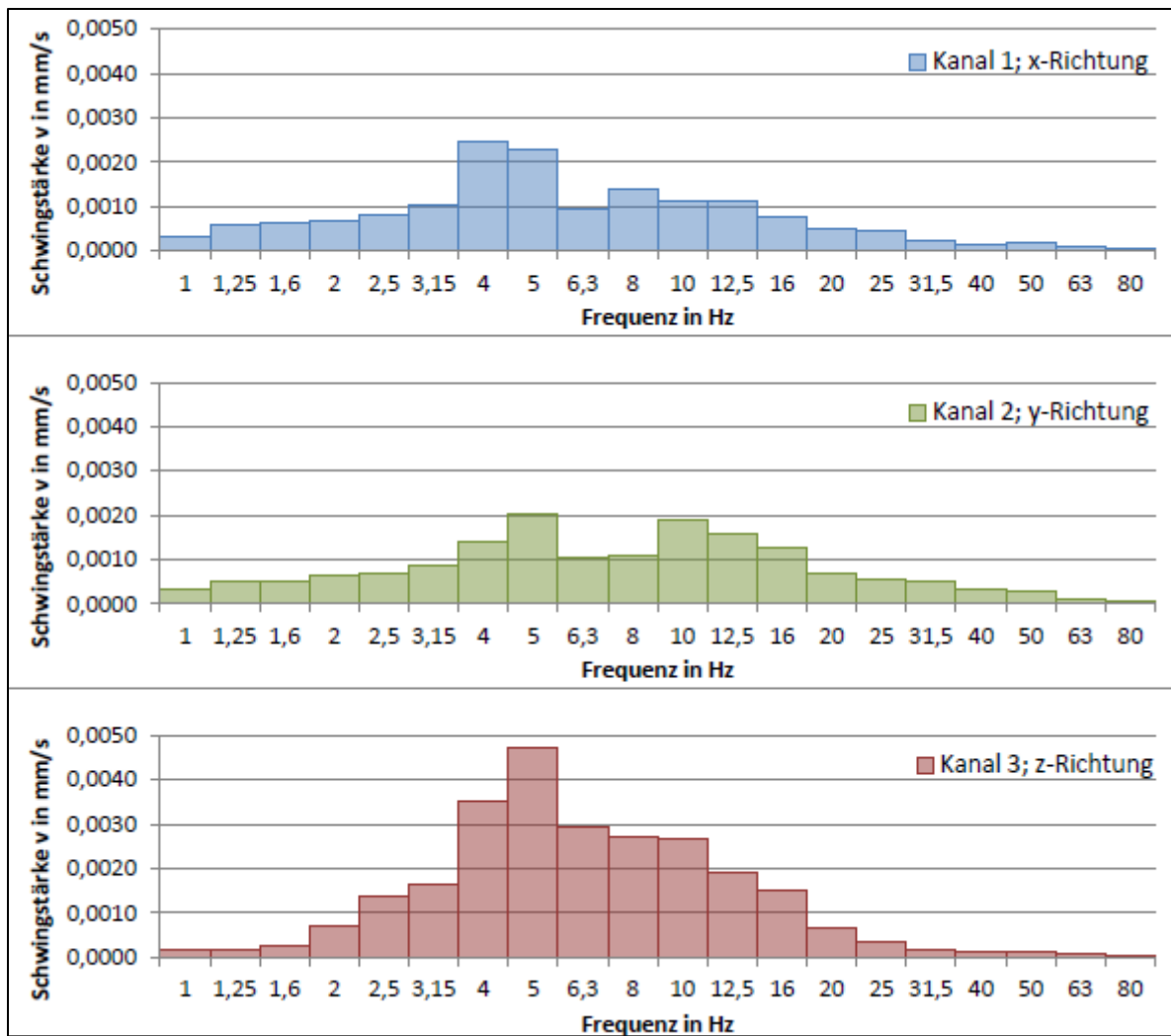
Abbildung 32: Terzspektrum zum Einzelereignis 8 (TÜV (2013))
