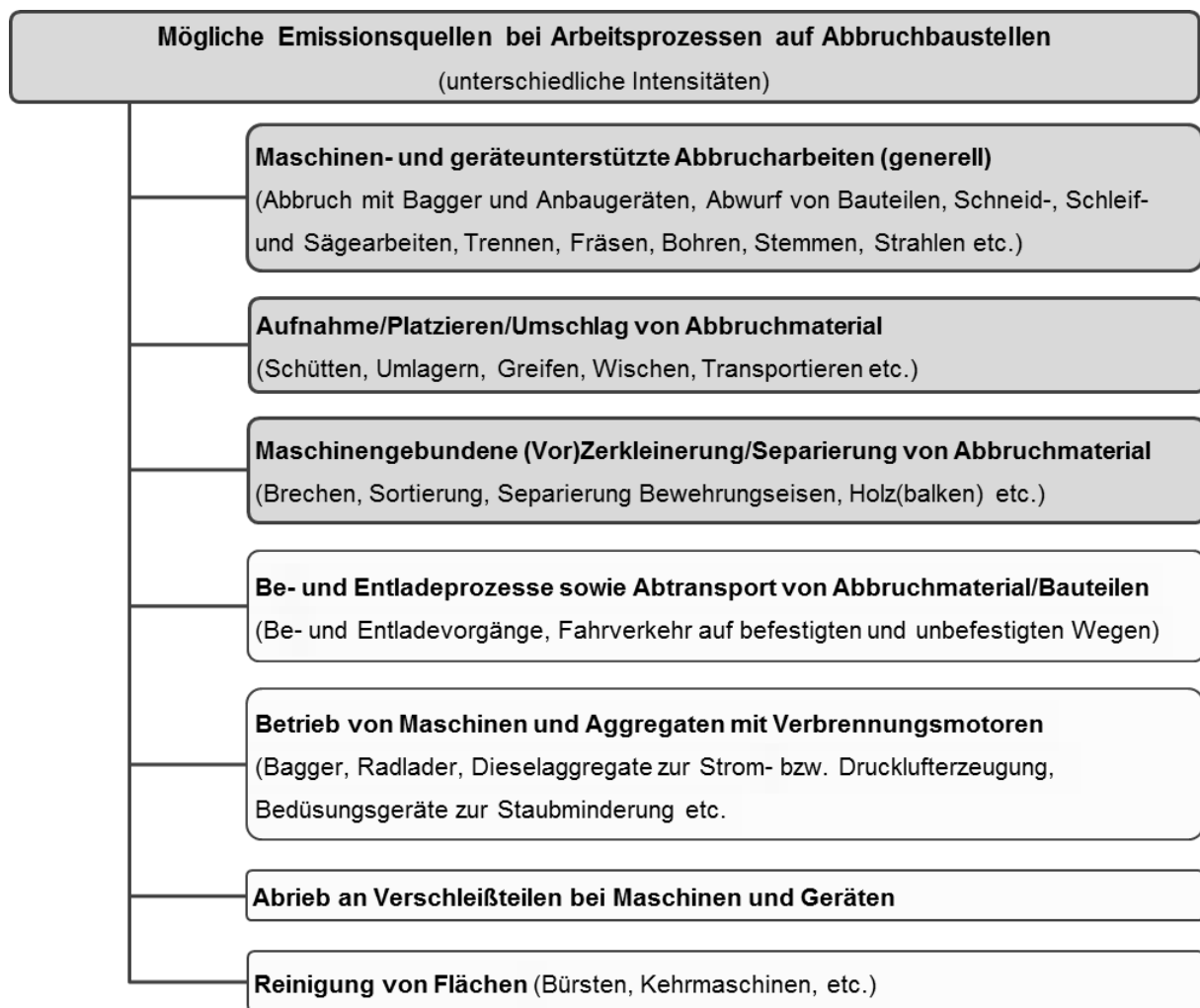
Abbildung 1: Mögliche Emissionsquellen bei Arbeitsprozessen auf Abbruchbaustellen
