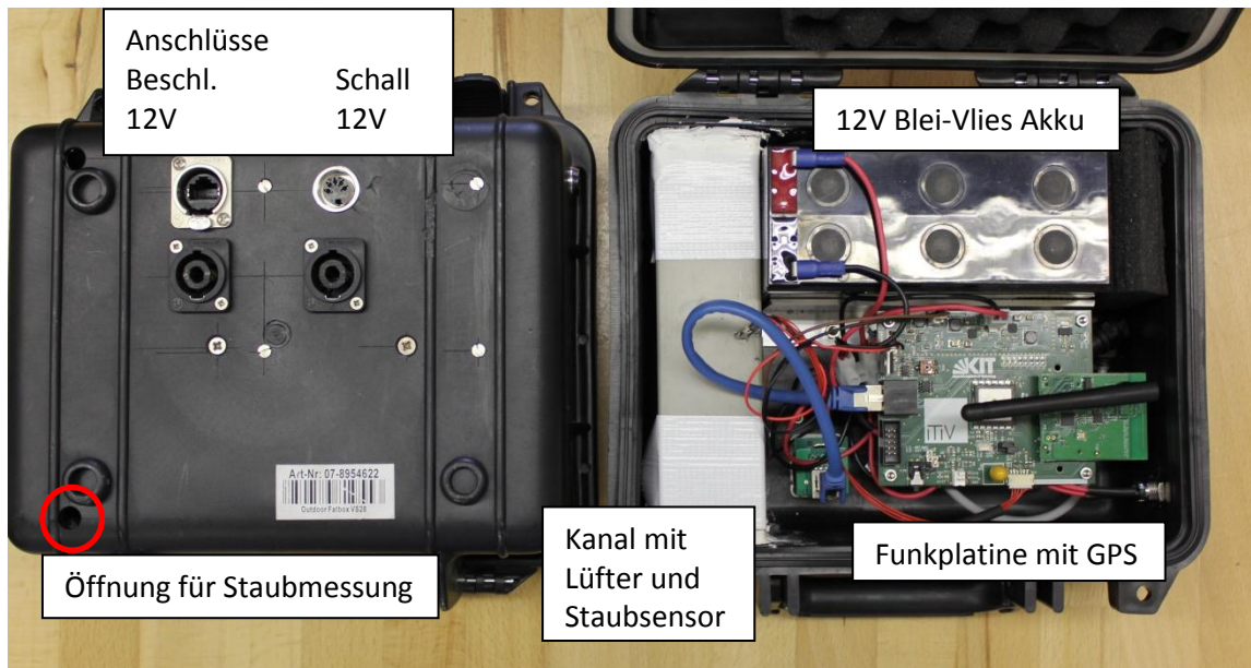
Abbildung 25: Messknotenelemente im Schutzkoffer – Unterseite mit Anschlüssen und Innenansicht
