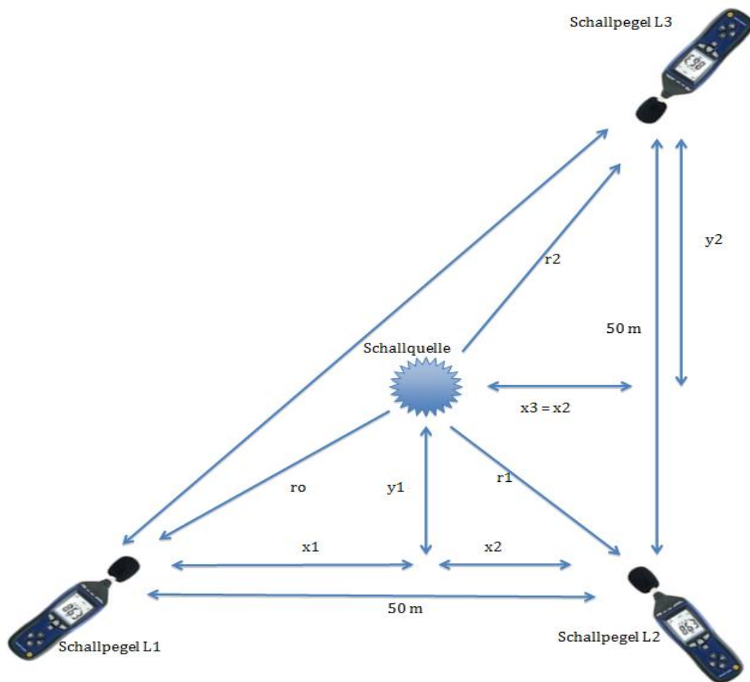
Abbildung 22: Lokalisation einer Schallquelle mit Hilfe von 3 Schallpegelmessgeräten
